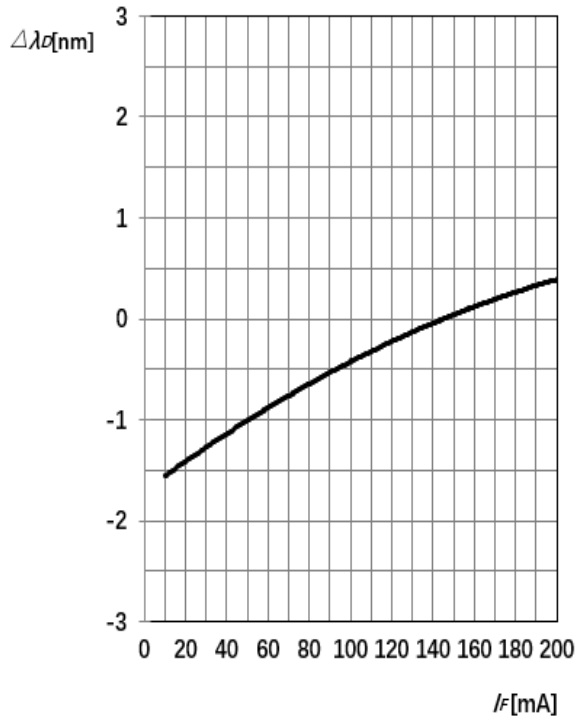
Fig 5. 波长偏移 Shift in Wavelength
