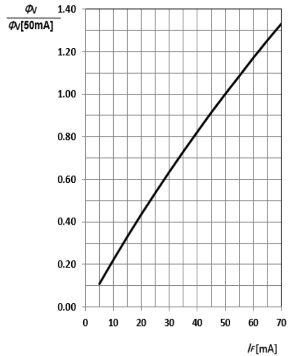
Fig 4. 相对发光强度 Relative Luminous Flux
