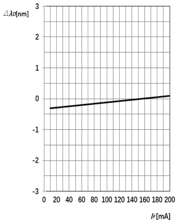
Fig 5. 波长偏移 Shift in Wavelength
