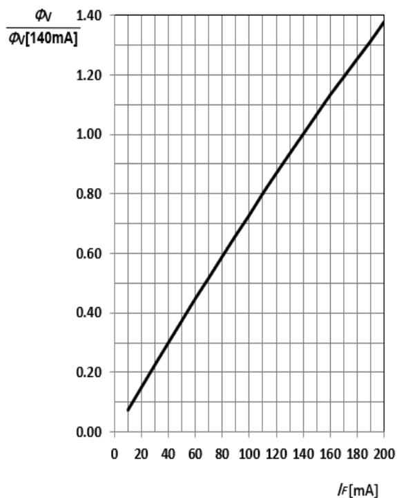
Fig 4. 相对发光强度 Relative Luminous Flux
