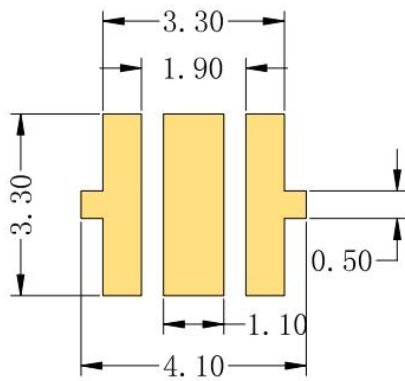
建议 PCB 焊盘
