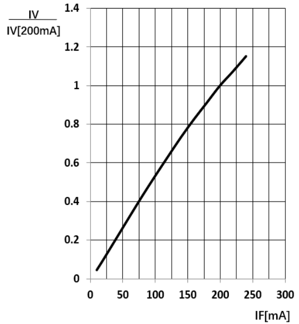
Fig 4. 相对发光强度 Relative Luminous Flux
