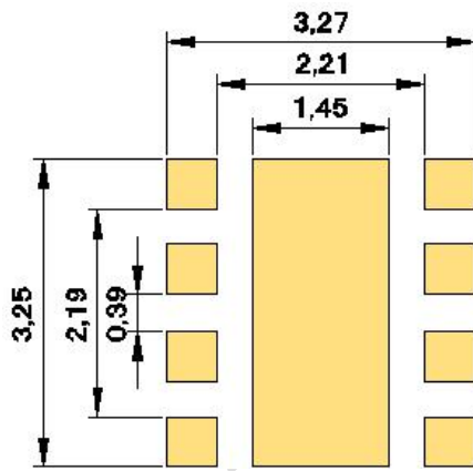
建议焊盘图
