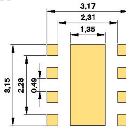
建议钢网图
