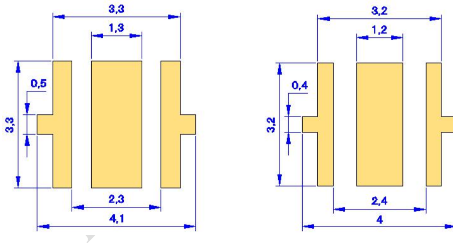
建议焊盘图
