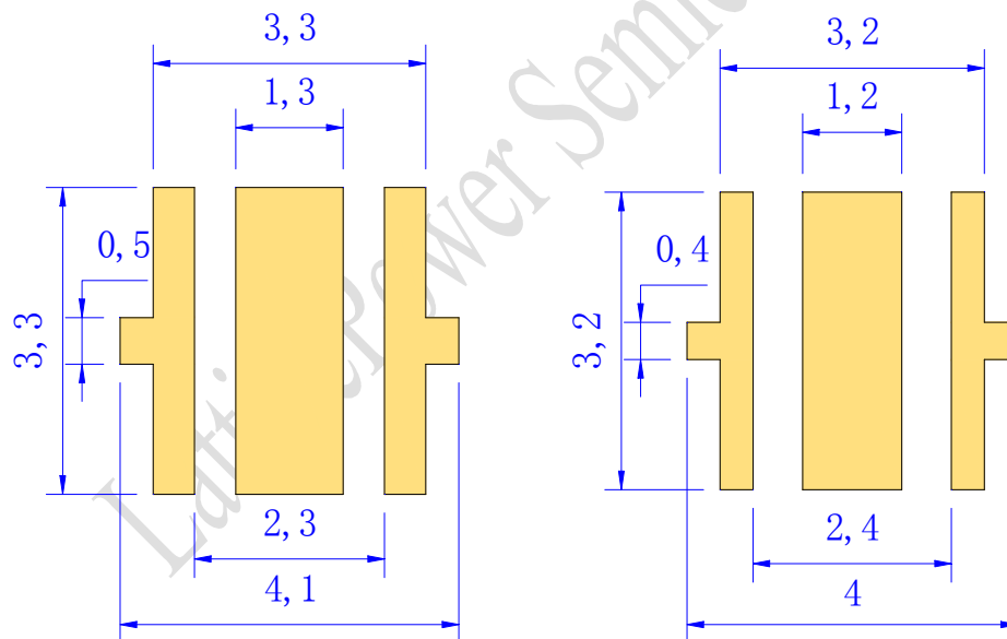
建议焊盘图
